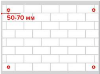
Рис. 4. Установка «маяков»
