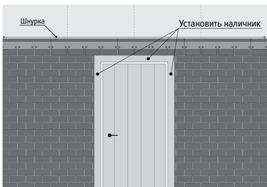
Рис. 9. Установка наличников
