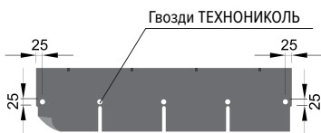
Рис. 3. Схема крепления фасадной плитки на 5 гвоздей
