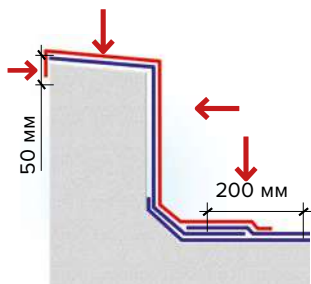
Кровля с наплавлением нижнего слоя
