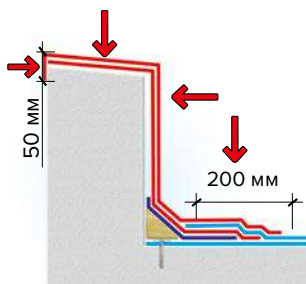
Кровля с мех. фиксацией
