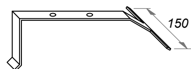
Крепежный элемент
