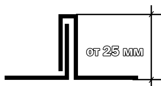
Рис. 3.27. Одинарный стоячий фалес
