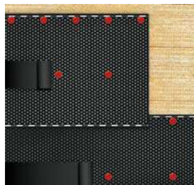
Рис. 3.43. Установка крепежа по центру материала Техноэласт ФИКС
