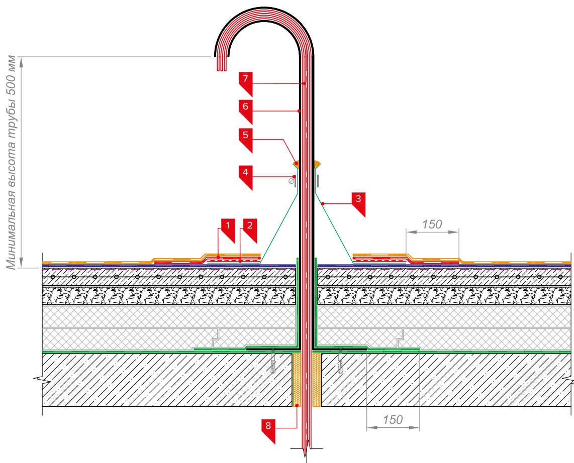
Рис. 3.38. Примыкание к гибким проходкам
