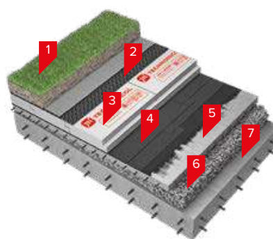
Рис. 1.6. Конструкция инверсионной озелененной крыши
