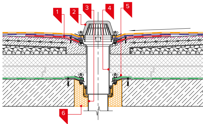
Рис. 3.51а. Примыкание к двухуровневой воронке
