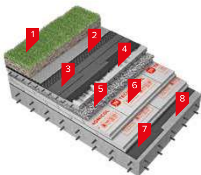
Рис. 1.5. Конструкция традиционной озелененной крыши
