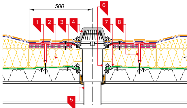
Рис. 3.51б. Примыкание к двухуровневой воронке
