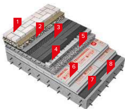
Рис. 1.3. Конструкция традиционной эксплуатируемой крыши под пешеходную нагрузку
