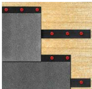
Рис. 3.44. Крепление полосы при устройстве однослойной кровли
