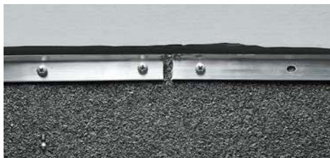
Рис. 3.21. Зазор между краевыми рейками
