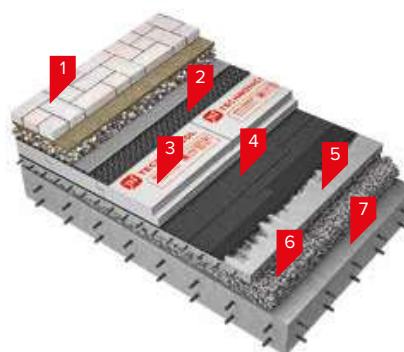
Рис. 1.4. Конструкция инверсионной эксплуатируемой крыши под пешеходную нагрузку
