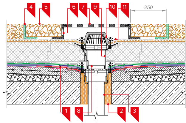
Рис. 3.53. Примыкание к воронкам в эксплуатируемых крышах
