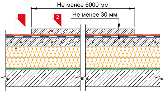
Рис. 4.1. Варианты устройства противопожарных рассечек 1. Утеплитель НГ и Г1; 2. Монолитная стяжка; 3. Утеплитель ГЗ-Г4
