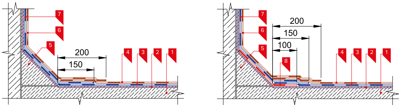
Рис. 3.18. Варианты раскладки водоизоляционного материала на переходном бортике при двухслойном водоизоляционном ковре. 1. основание под кровлю; 2. Праймер битумный ТЕХНОНИКОЛЬ №01; 3. нижний слой водоизоляционного ковра; 4. верхний слой водоизоляционного ковра; 5. переходной бортик; 6. верхний слой водоизоляционного ковра на вертикальной поверхности; 7. нижний слой водоизоляционного ковра на вертикальной поверхности; 8. слой усиления
