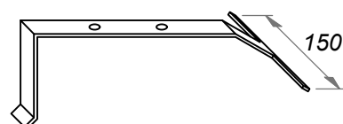
Крепежный элемент
