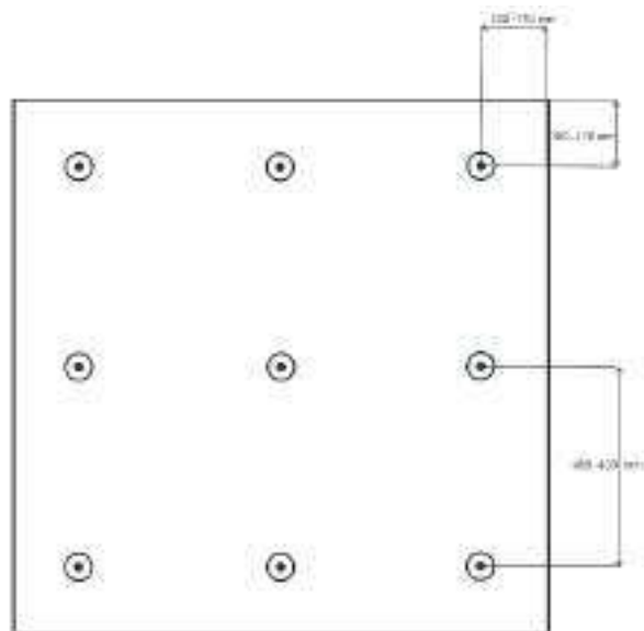
Схема установки крепежных элементов для плит размером 1200 x 1200 мм
