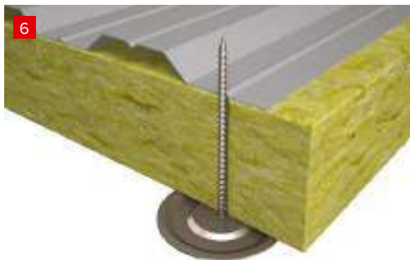
Закрепление плиты ТЕХНО ОЗМ при помощи самосверлящих винтов с шляпкой
